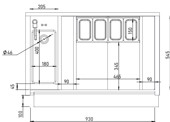
WHS 100 LATO / SIDE
