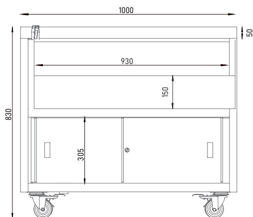
WHS 100 FRONTE / FRONT
