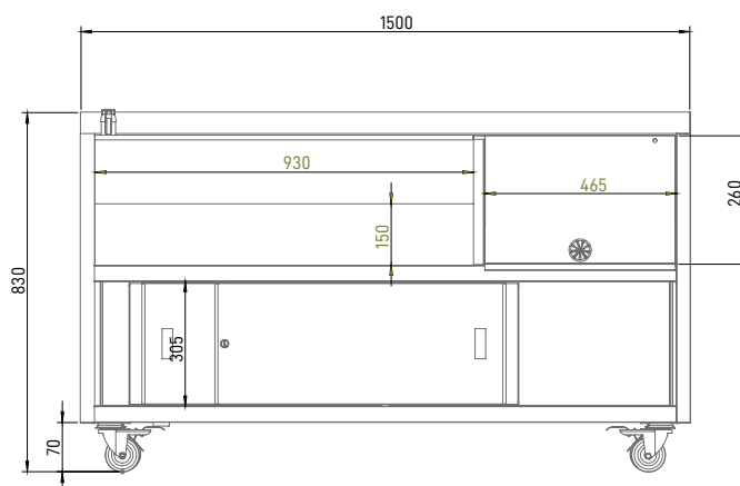
WHS 150 FRONTE / FRONT
