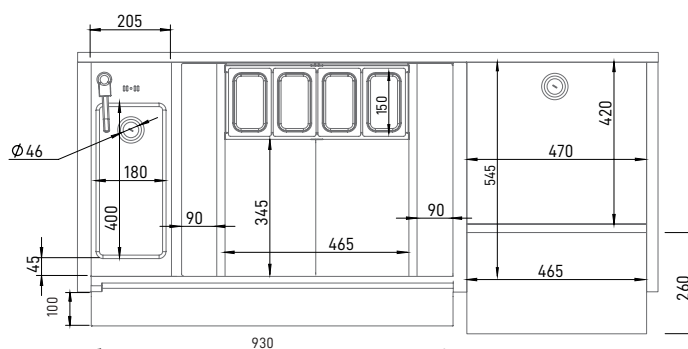
WHS 150 LATO / SIDE
